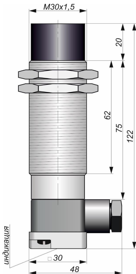
Габаритный чертеж
